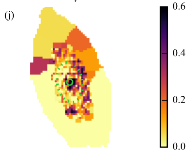
v_{\star} [ \text{km s}^{-1} ]
