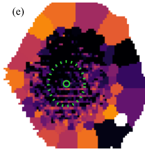
b^{\text{loc}}
