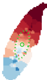
v_{\star} [\text{km s}^{-1}]
