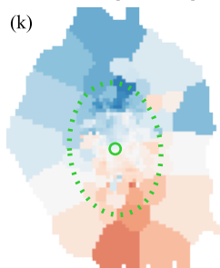
v_{\star} [ \text{km s}^{-1} ]
