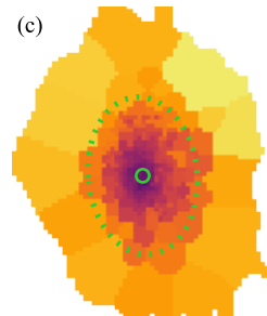
\log \Sigma_{\star} [ M_{\odot} \text{ pc}^{-2} ]
