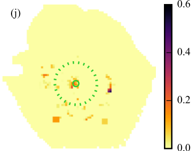
\tau_{\text{V}}
