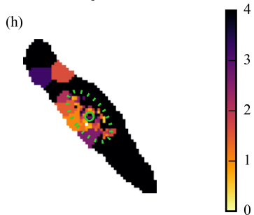
v_{\star} [ \text{km s}^{-1} ]
