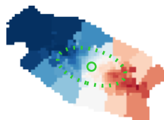
v_{\star} [\text{km s}^{-1}]
