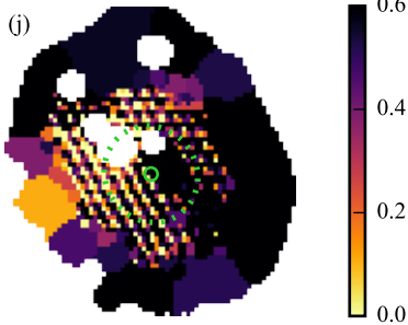
\tau_{\text{V}}
