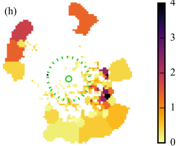
v_{\star} [\text{km s}^{-1}]
