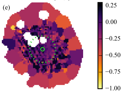
b^{\text{loc}}
