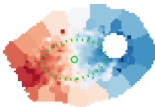
v_{\star} [ \text{km s}^{-1} ]
