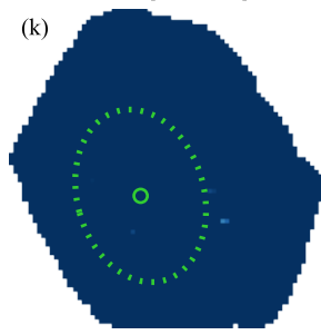
v_{\star} [\text{km s}^{-1}]
