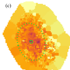
\log \Sigma_{\star} [\text{M}_{\odot} \text{pc}^{-2}]
