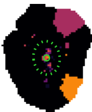
v_{\star} [\text{km s}^{-1}]
