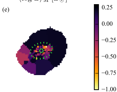
b^{\text{loc}}
