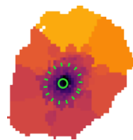
\log \Sigma_{\star} [M_{\odot} \text{pc}^{-2}]
