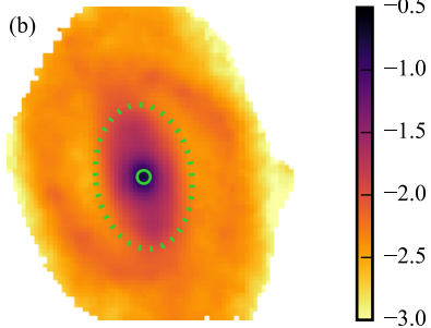
\langle \log Z \rangle_{\text{M}} [\text{Z}_{\odot}]
